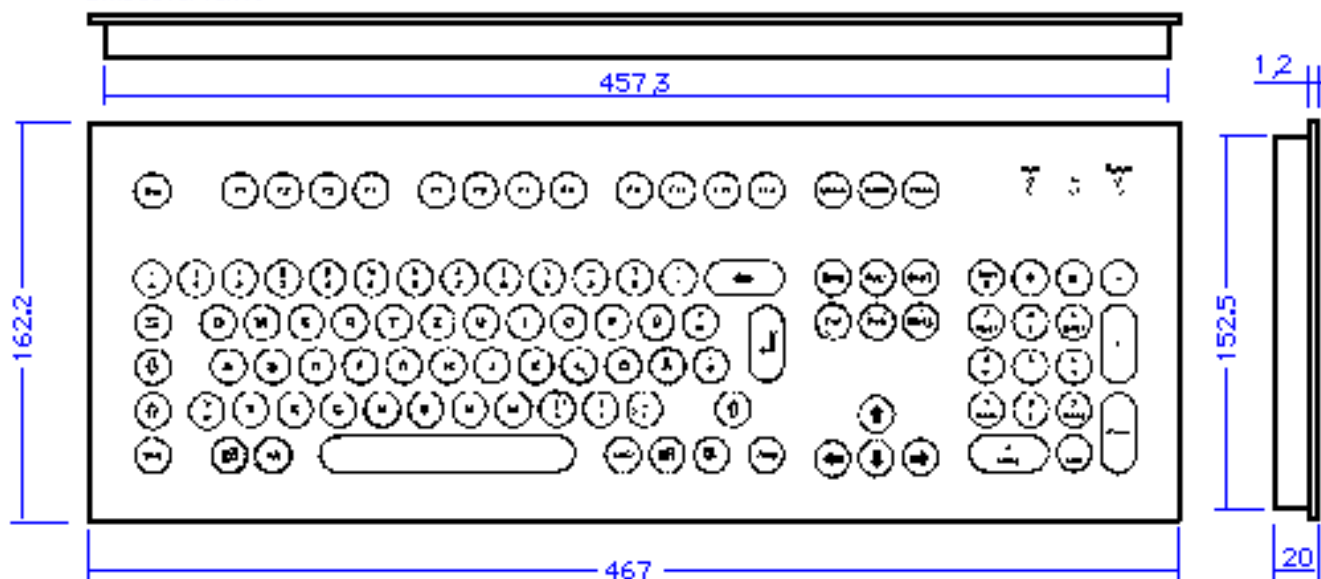
Einbauvariante
