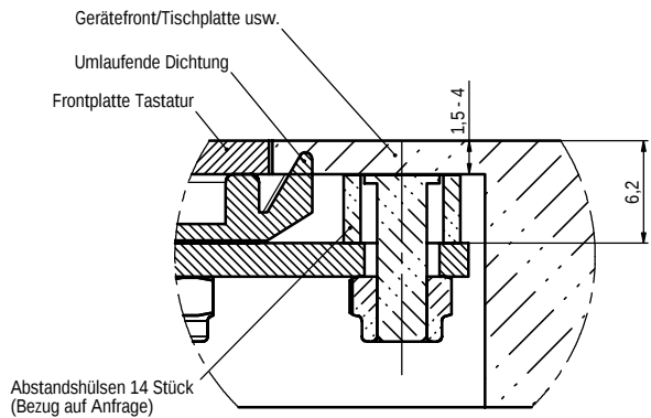
Einbauvorschlag Schnitt A-A (4 : 1)
