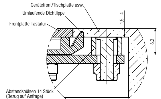
Einbauvorschlag Schnitt A-A (4 : 1)
